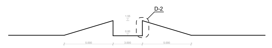
Lõige 1-200
