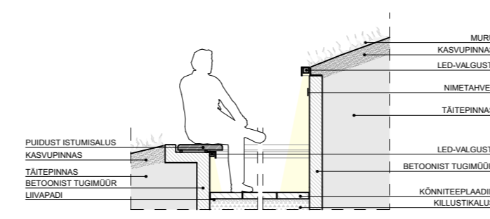
D-1 1-50
