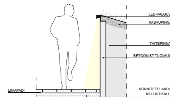
D-2 1-50
